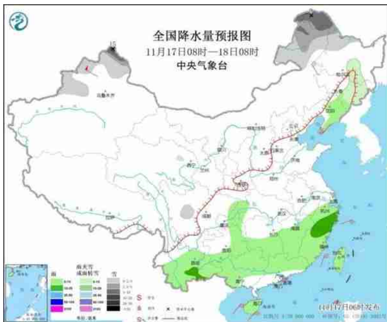
图2 全国降水量预报图(11月17日08时-18日08时)
